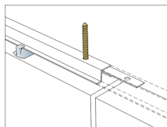
Infästning av Skarvbleck för Baffleprofil
