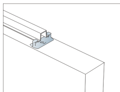
Bafflarna säkras med ett clips
