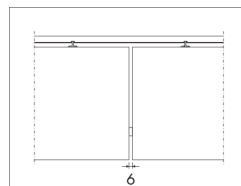
Styrstiftet ger ett distinkt mellanrum 6 mm mellan bafflarna
