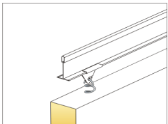
Detalj av nedpendling (M124_det2)
