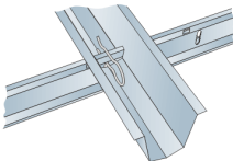
Möte mellan profiler med Sprint
