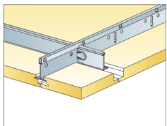
Tvårprofiler används för att hålla plattorna i position
