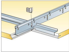
Möte mellan Huvudprofil och Förstärkningsprofil
