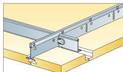
Tvårsprofil används för att hålla plattorna i position
